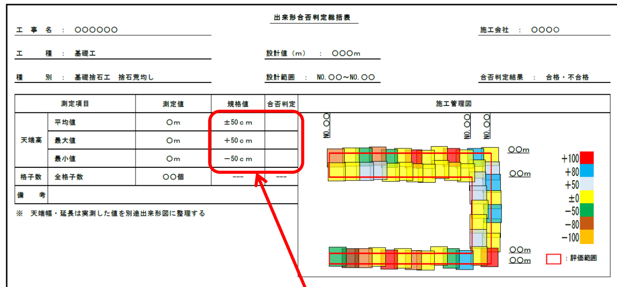
図- 5.2 出来形管理図 (荒均し) (例)
