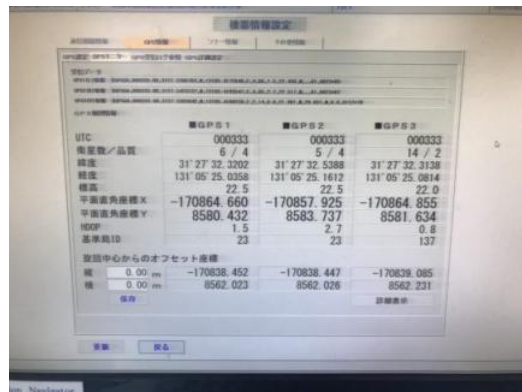
施工管理システムによるGNSS受信座標
