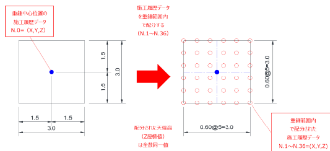
図- 4.4 施工履歴データ分配図(例)
