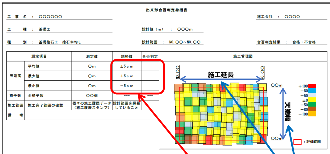
図- 5.1 出来形管理図 (本均し) (例)
