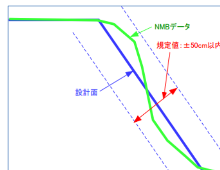
図-3.5 法面の法線方向の差分
