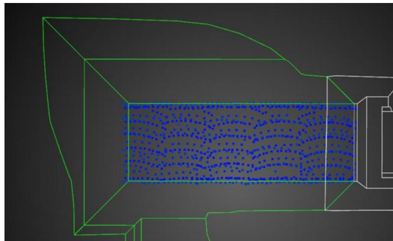
施工履歴データ取得例
